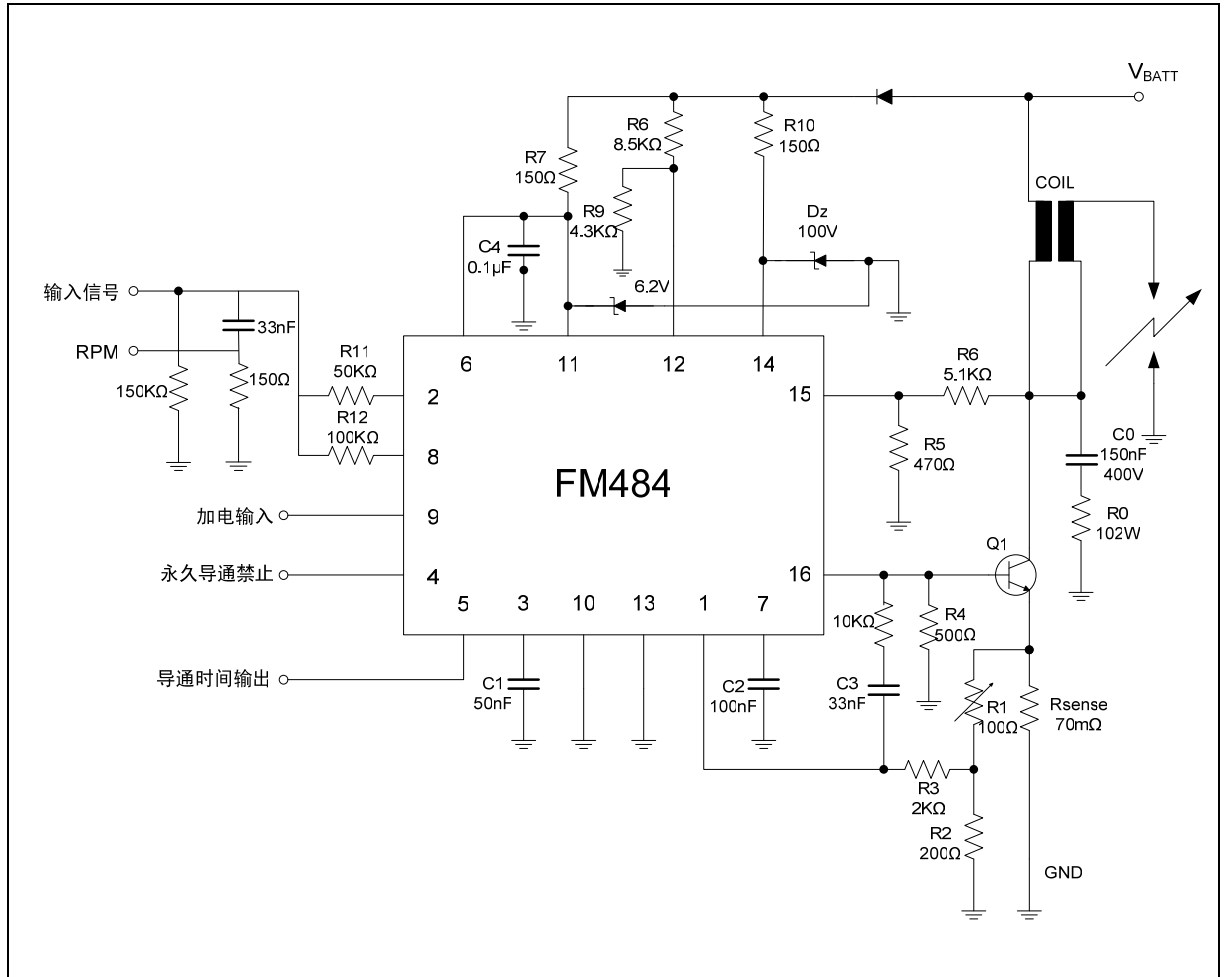
图 3-1 FM484 应用电路图
