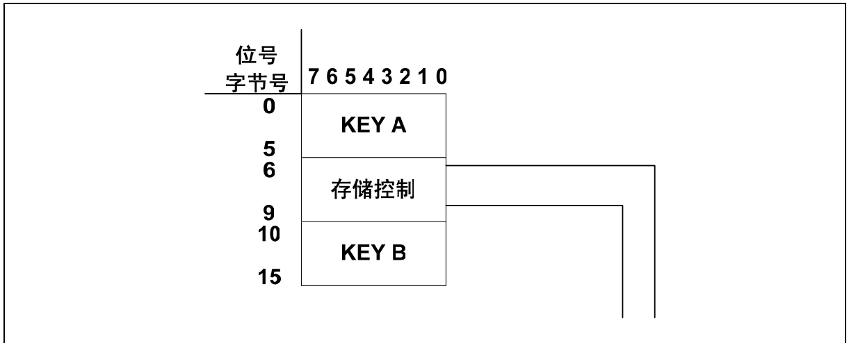
图 5-2 FM11RF08 存储器块 3 结构图
