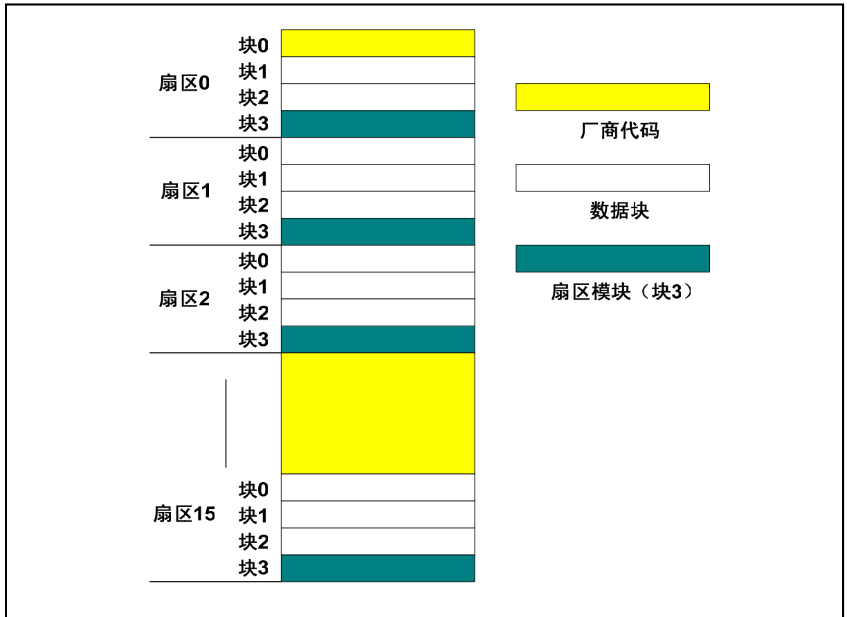
图 5-1 FM11RF08 存储器分区图
