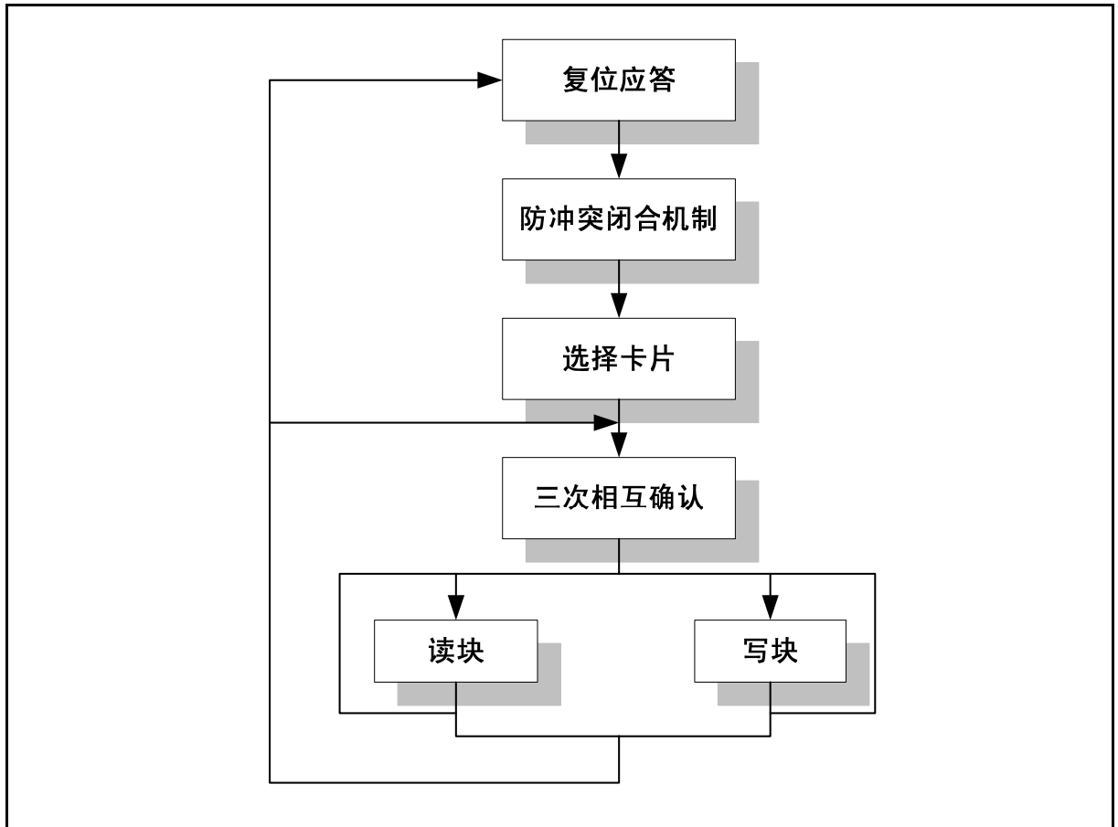
图 4-1 FM11RF08 交易流程图
